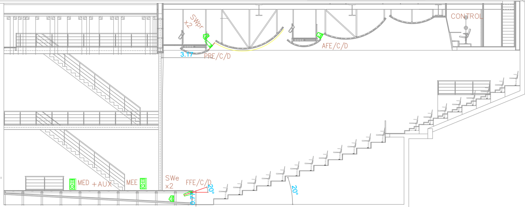
TEATRE PLAZA CASTELLSDEFELS Distribució altaveus alçat
